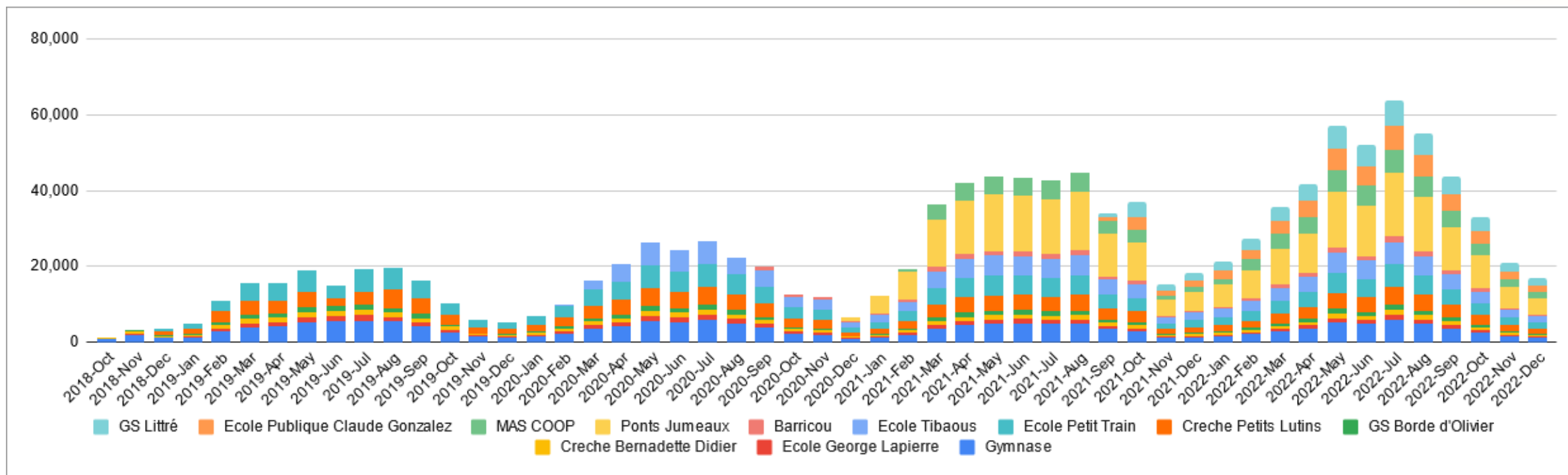
Production par station (kWh)
